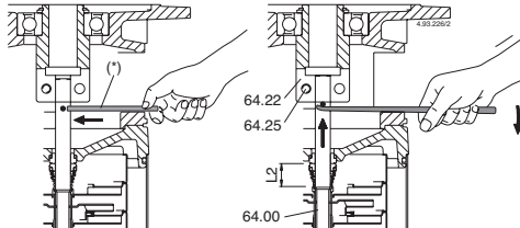
Abb. 6a Stehender Läufer, Welle nicht blockiert in Kupplung (*) Stift für Wellenanheben.
