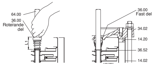
Fig. 5 Montering av axeltätning
