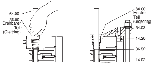
Abb. 5 Montage Gleitringdichtung
